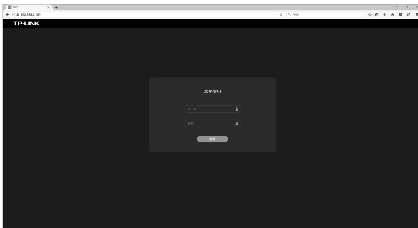
图5-2 登录界面
